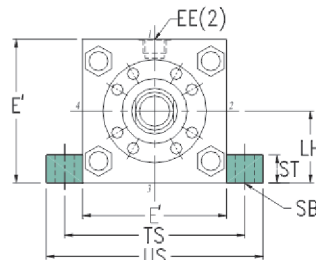
Side Lugs (ISOMS2)
